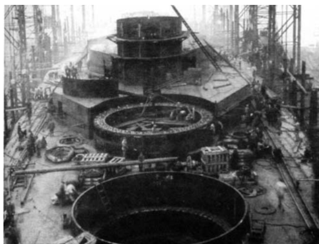
Корпус линкора "Хьюга" на стапеле. 1916 г.
