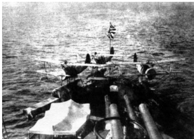
Кормовая оконечность линкора "Исе" с установленными на ней катапультами и гидросамолетами
