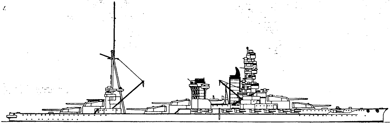
Линейный корабль "Исе". 1930 г. (Наружный вид)
