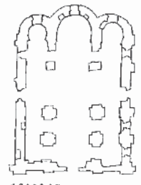
1 0 1 2 3 4 5 М План. Микло-Дворецкий собор в Н. Новгороде
