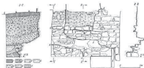
Рис. 2. Церковь. План в Онихах. Шурф у северо-западного угла. А — верхняя граница кладки 1127 г.; В — то же конца XII в.; С — то же до XIV в.; УГВ — уровень грунтовой воды; 1 — дверь; 2 — земля со строительными мусорами; 3 — древний строительный раствор с фресками и инкрустацией; 4 — древний строительный раствор с землей; 5 — строительный мусор; 6 — кирпичный конструктивный слой; 7 — черная земля
