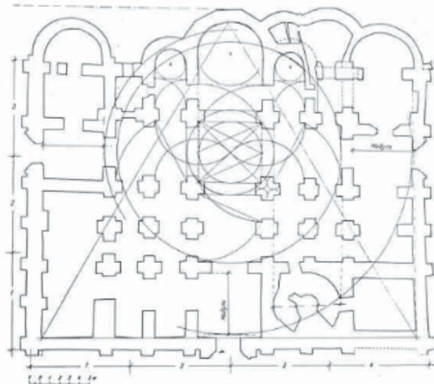
Сетка пропорций плана Софийского собора в Новгороде.
