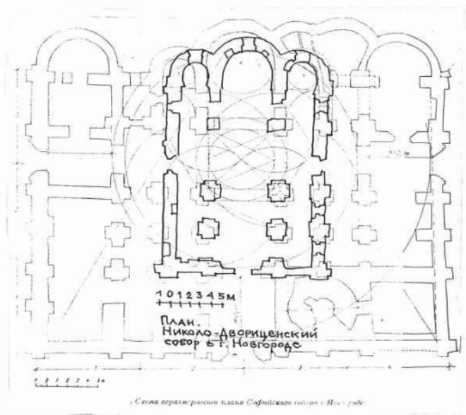
РИС.8: Наложение планов Софийского собора в Новгороде и Николо-Дворищенского собора в Новгороде.
