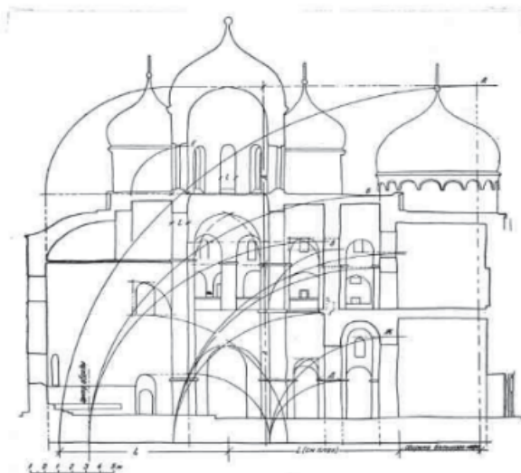
Схема соотношения продольного разреза Софийского собора в Новгороде.
