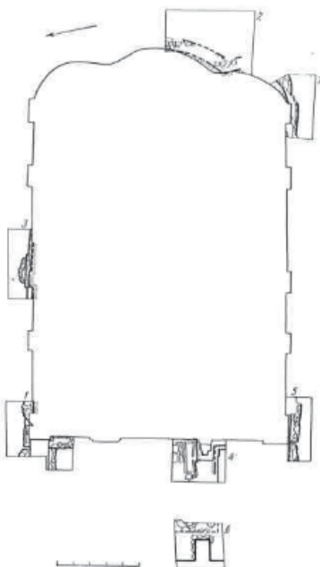
Рис. 1. Церковь. План в Онихах. План расположенных участков здания: 1-7 — расположенные шурфы
